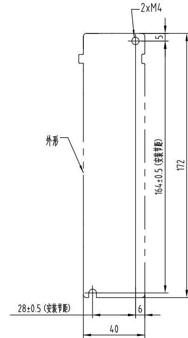
安装孔加工图
