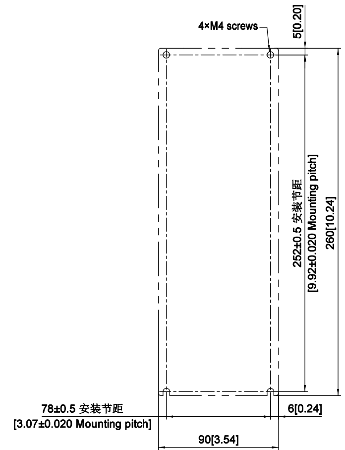
安装孔加工图 Mounting Hole Diagram
