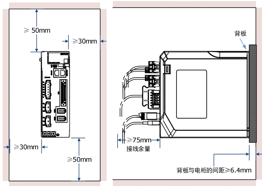
图 2-2 安装单个驱动器至控制柜时
