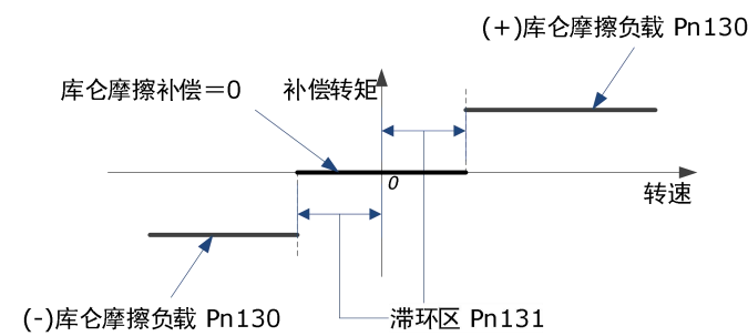
图 8-27 摩擦补偿示意图
