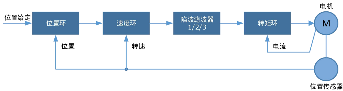
图 8-30 陷波滤波器工作示意图
