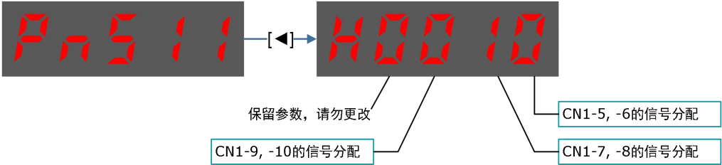
图 5-3 轴一输出信号分配示意
