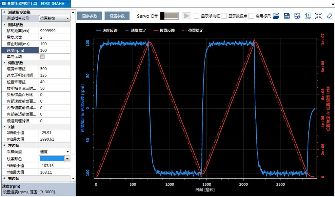
图 8-21 “位置斜坡” 指令采样结果的示例
