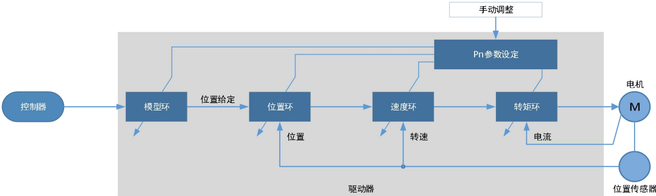
图 8-29 模型跟踪控制的示意图
