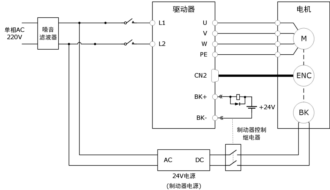
图 3-4 制动器接线示例
