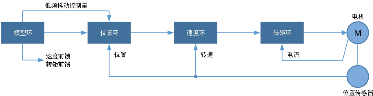
图 8-34 低频振动抑制工作示意图
