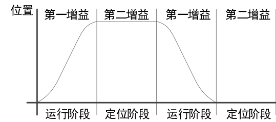
图 8-23 增益切换示例
