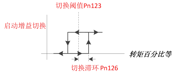
图 8-25 切换滞环示意图
