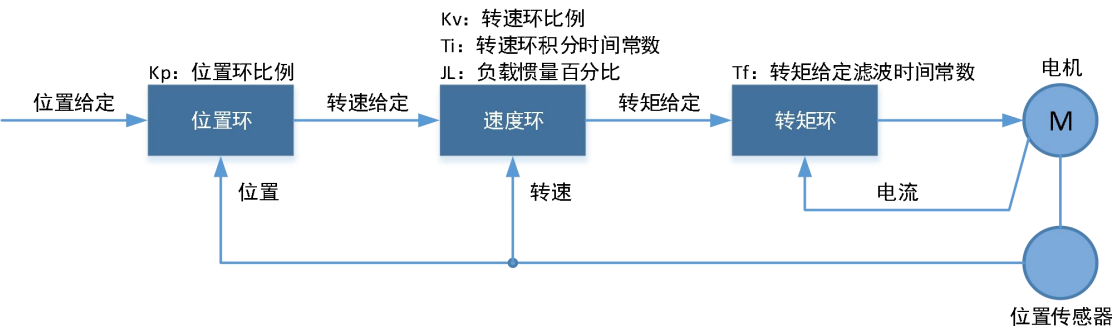
图 8-2 伺服控制原理
