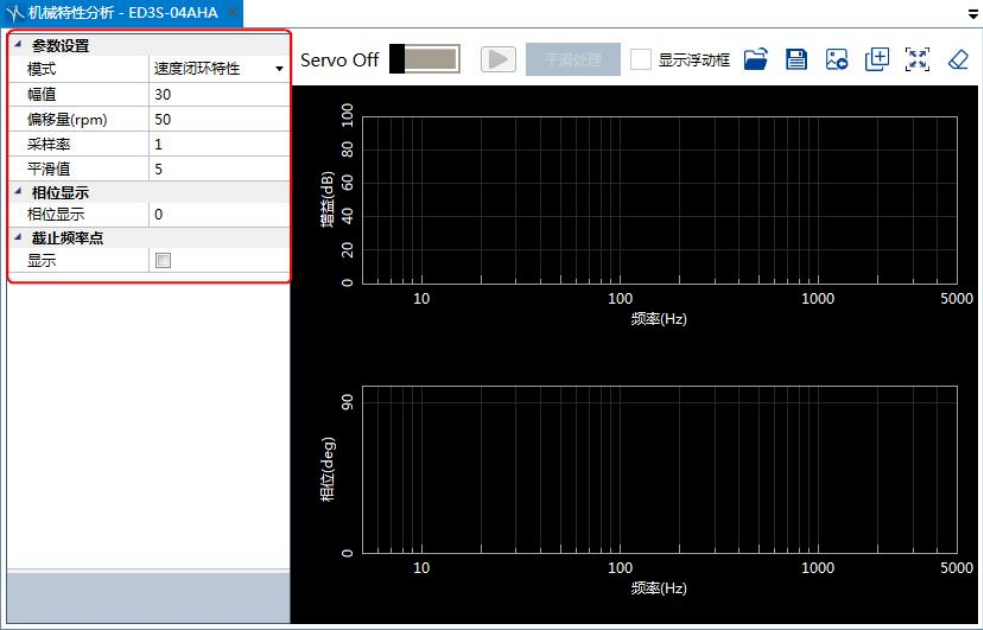
图 8-44 设置参数
