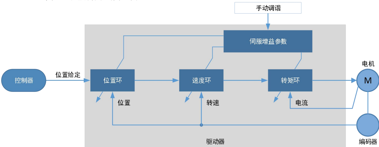
图 8-6 手动调谐的工作示意图
