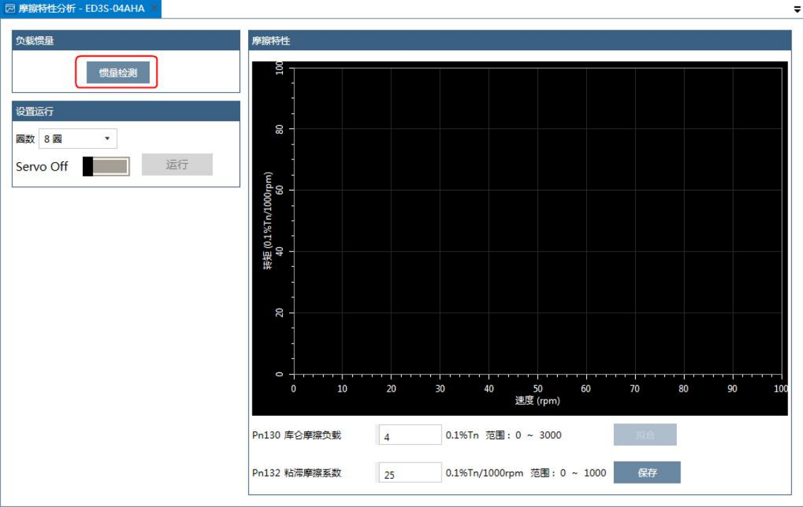
图 8-55 执行惯量检测操作
