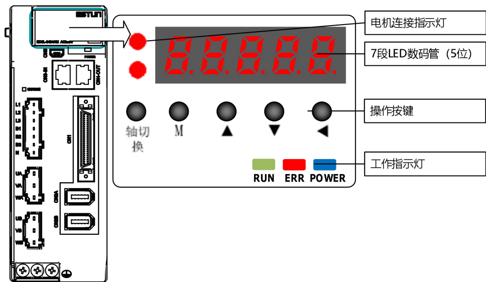
图 4-1 操作面板图示
