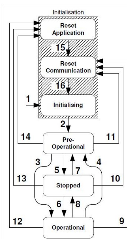
网络管理状态转换图
