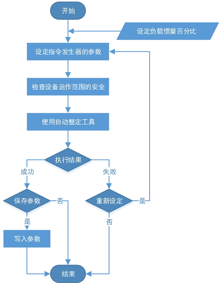
图 8-10 自动整定工具的使用流程
