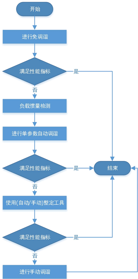
图 8-3 调整流程
