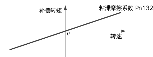
图 8-28 粘滞摩擦与转速的关系
