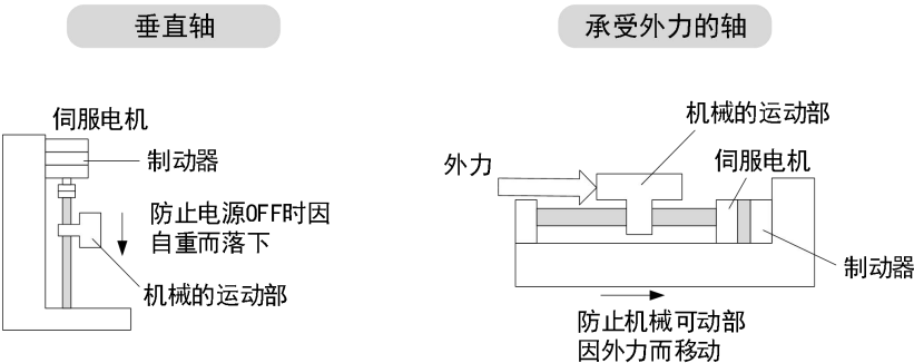
图 3-3 带制动器电机的应用示意图
