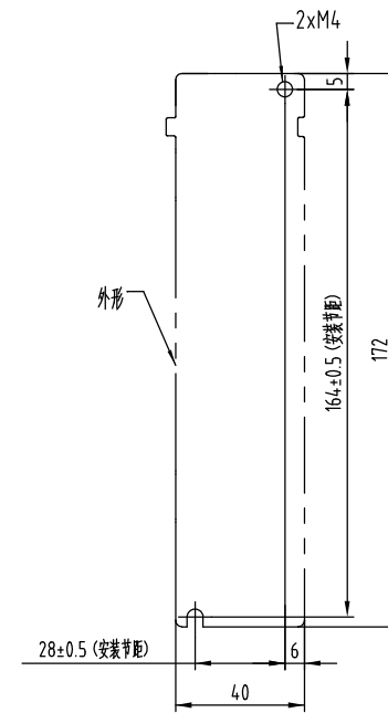
安装孔加工图
