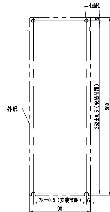
安装孔加工图 单位: mm
